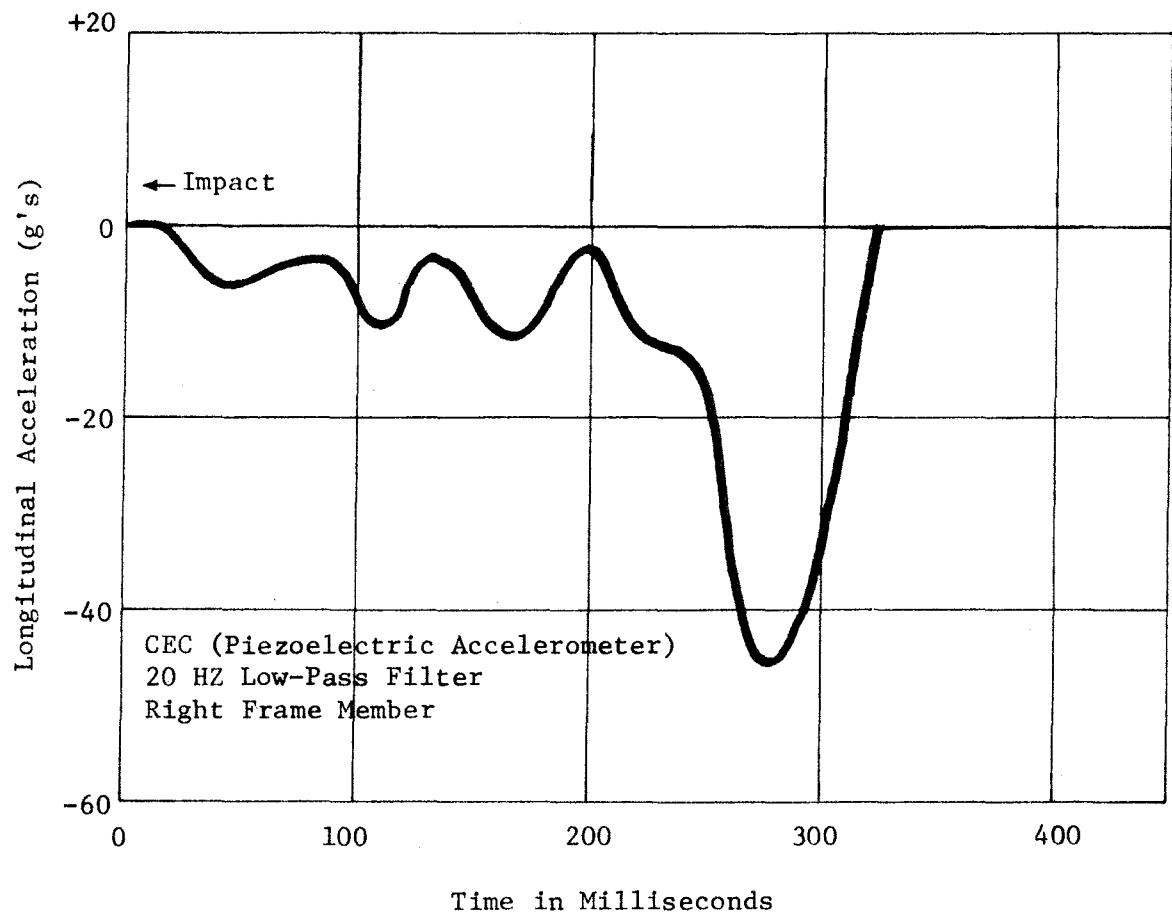
Figure A1, Longitudinal Accelerometer Data, Test 505 B-A.
