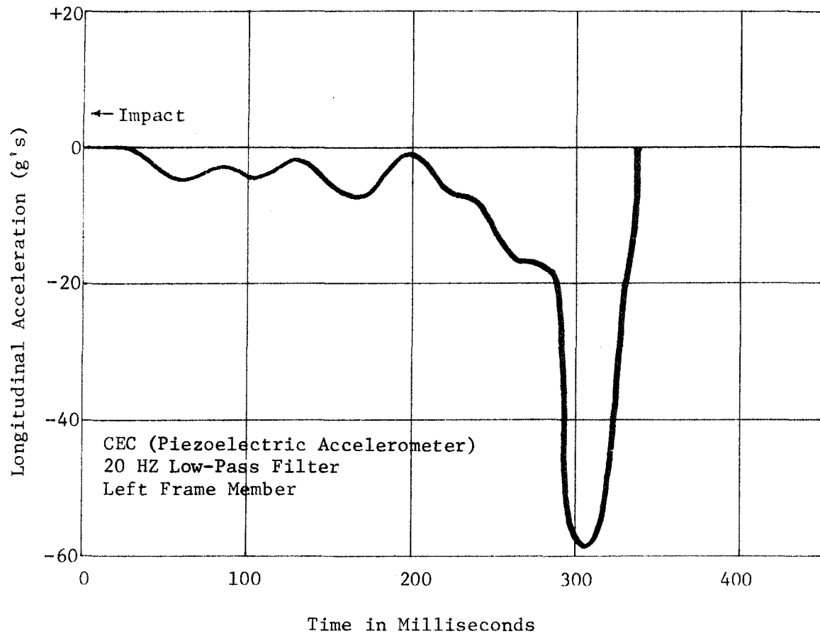
Figure A2, Longitudinal Accelerometer Data, Test 505 B-A.
